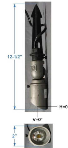
FIG. 1 LUMINAIRE
